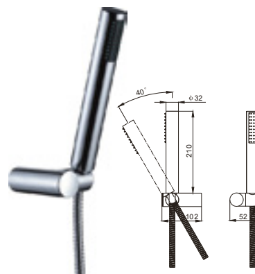
Supporto in plastica con rosone per doccetta "Queen"
